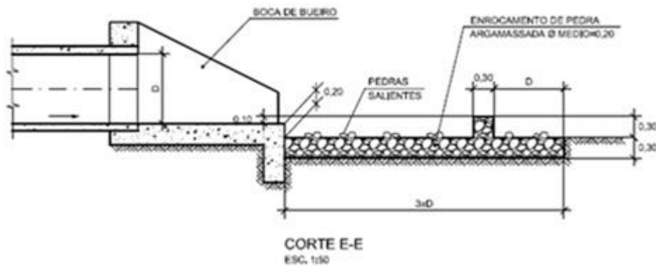
1891 Ilustração 8.4- Dissipador.
