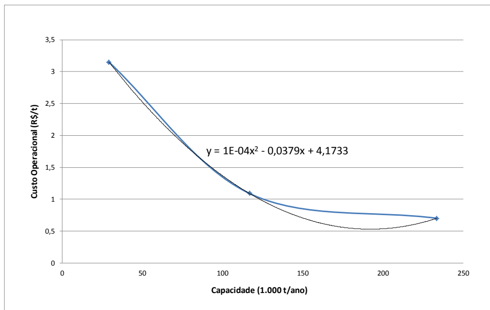
2190 Gráfico 9.4 – Variação do custo operacional da CB em função da capacidade
