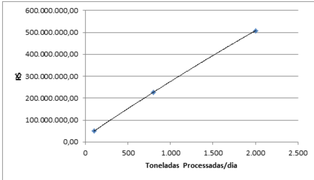
2151 Gráfico 9.1 – Variação do custo de implantação do ATS em função da quantidade de resíduos 2152 processados 2153 por dia 2154
