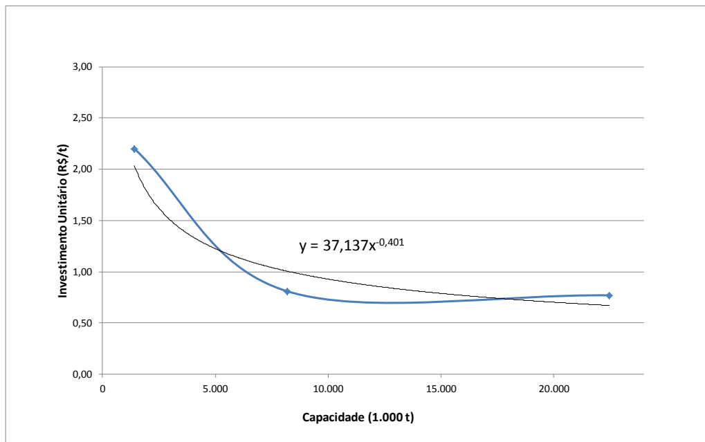
2209 Gráfico 9.5 – Variação do custo da implantação do ARCC em função da capacidade
