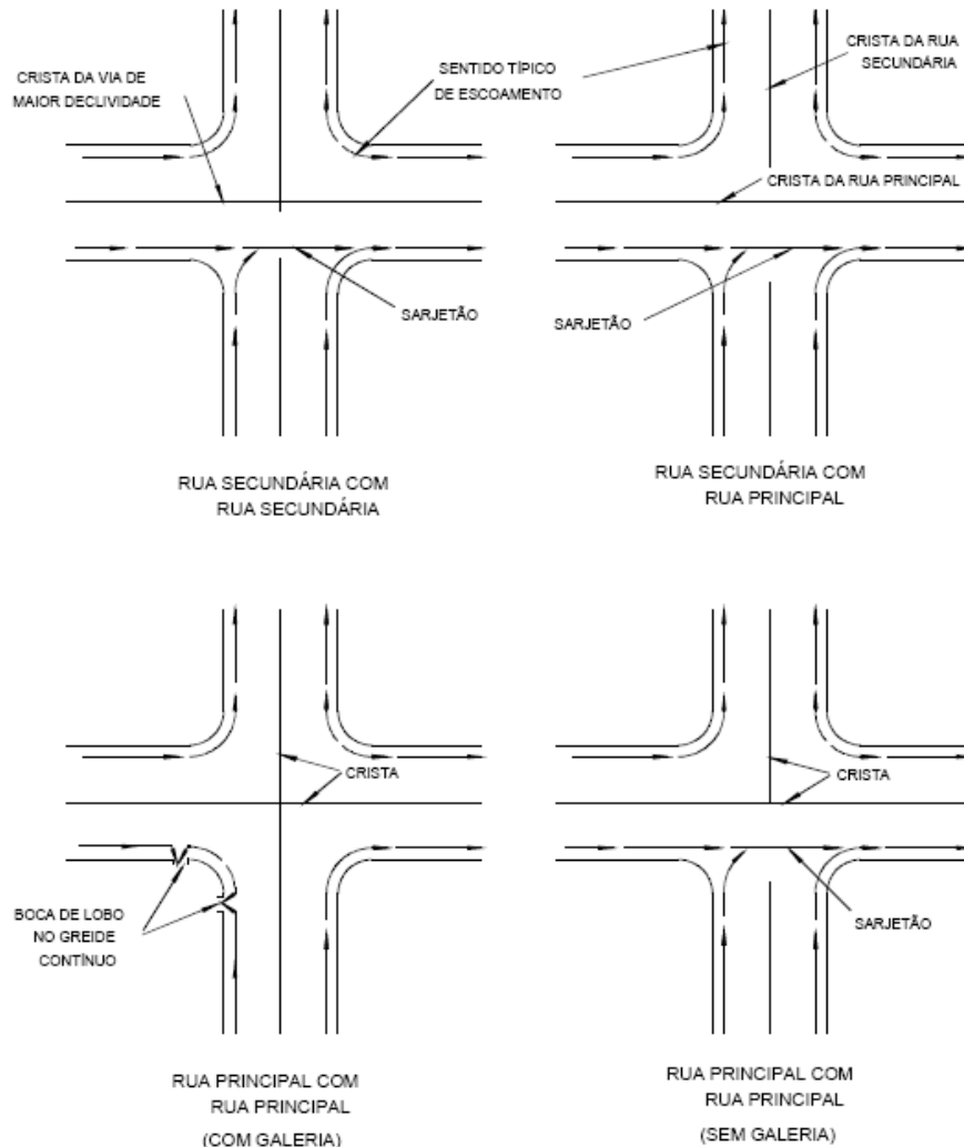
5389 5390 Figura 4.2: Configurações típicas de cruzamentos em sistema de drenagem 5391
